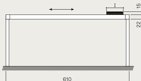
Massimo ingombro lame compattate Lama: H 2 cm - Ingombro max: 80 cm Lama: H 3 cm - Ingombro max: 110 cm
