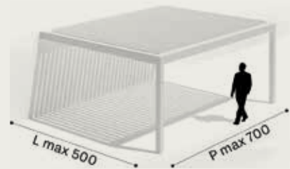
Pergola addossata a muro lato profondità Pergola leaning against a wall, depth side
